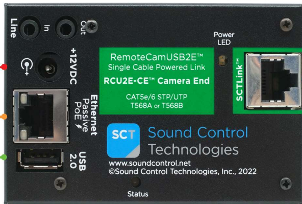
RCU2E-CE™
